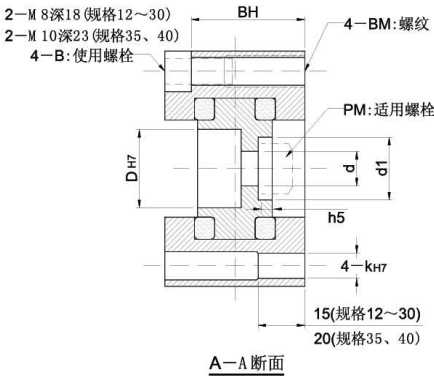
A-A 断面
