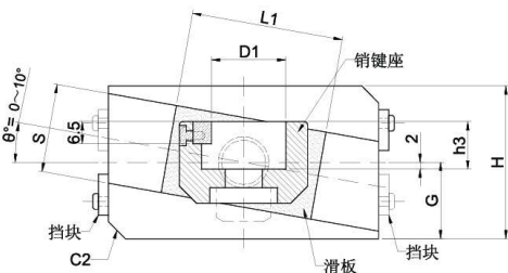
B-B 断面
