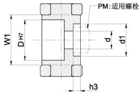
A-A 断面
